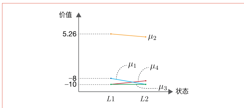
图 2-17 各策略的状态价值函数的图形
