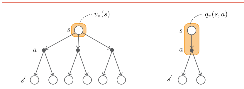
图 3-11 状态价值函数的回溯线形图（左）与 Q 函数的回溯线形图（右）
